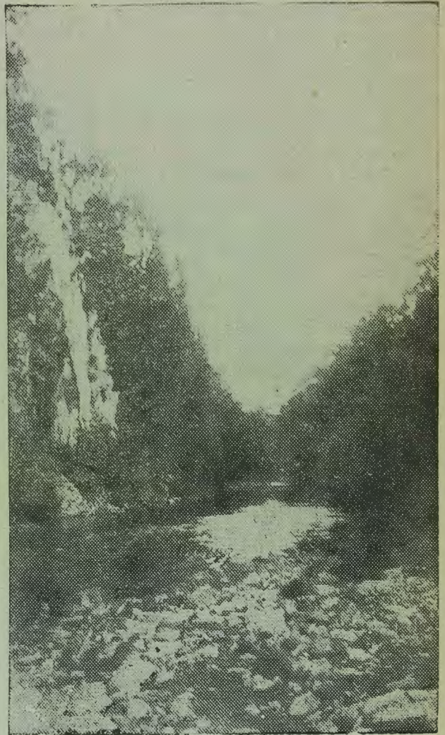
Ев. АО. „Белая скала“—обнажение мрамора.
